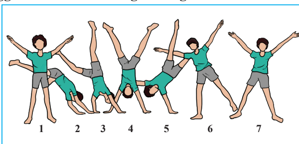
Gambar 6.4 Gerak meroda
