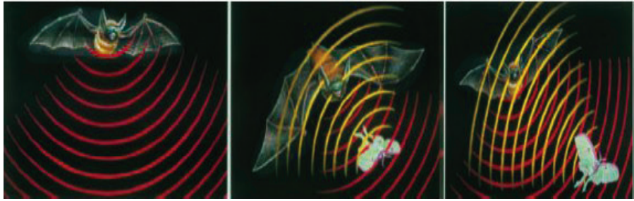
Gambar 10.18 Ekolokasi Kelelawar
