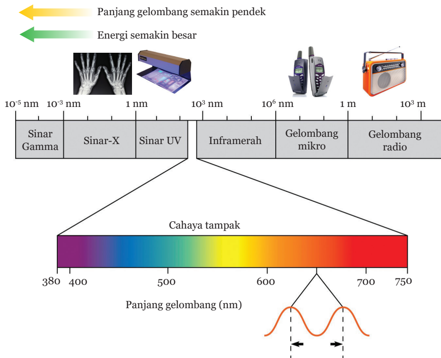
Gambar 11.8 Spektrum Elektromagnetik
