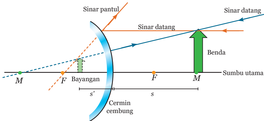
Gambar 11.20 Pembentukan Bayangan pada Cermin Cembung, Bayangan yang Terbentuk Bersifat Maya dan Tegak
