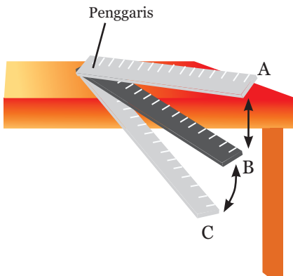
Gambar 10.7 Penggaris Plastik yang Digetarkan
