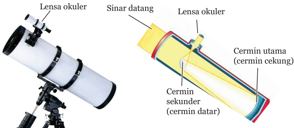
Gambar 11.42 Teleskop Pantul
