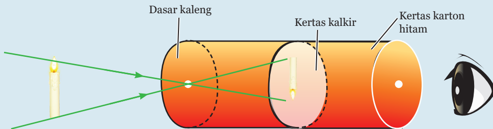
Gambar 11.35 Skema Kamera Obscura
