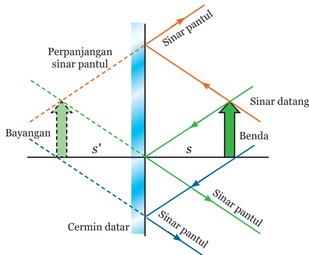
Gambar 11.10 Pembentukan Bayangan pada Cermin Datar
