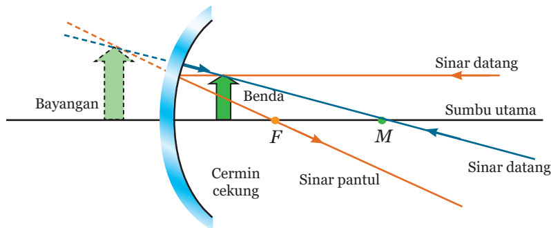
Gambar 11.17 Pembentukan Bayangan jika Benda Berada di Antara Titik Fokus dan Cermin Cekung
