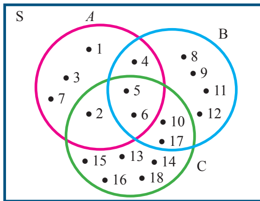
Gambar 2.16 Diagram Venn himpunan A , B , dan C
