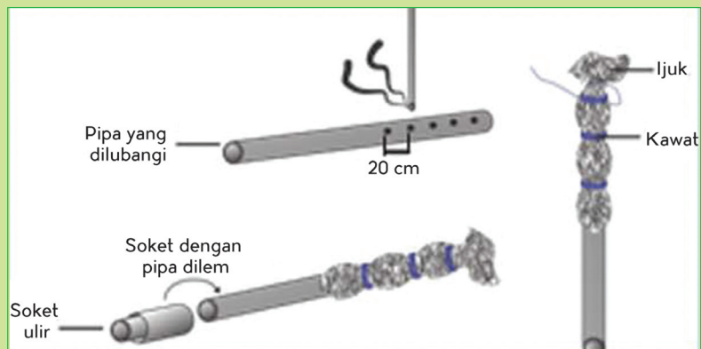
Gambar 2.9. Pipa penyaring
